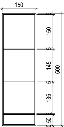
Base da Torre Vista Frontal
