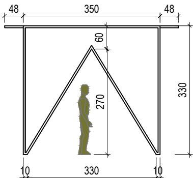
Bandeirola - Portal Vista Frontal
