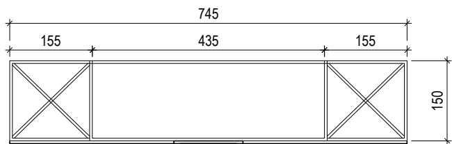
Vista Superior
