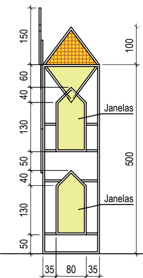
Vista Lateral
